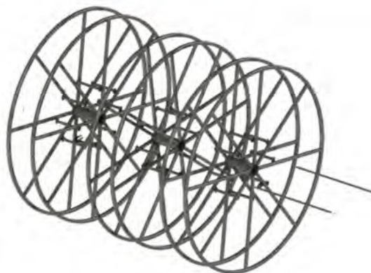
Touret - Vue éclatée
